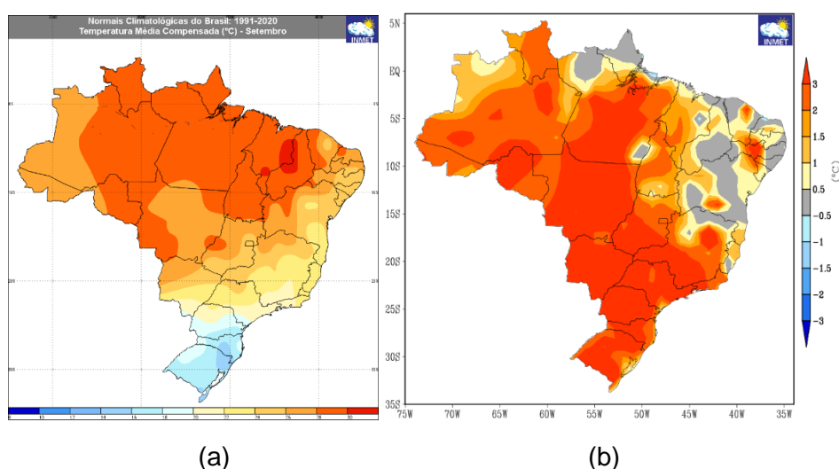
Figura 1 – (a) Climatologia no mês de setembro (1991 - 2020) e Desvio em setembro de 2023 da temperatura média do ar, expressa em °C. Fonte: INMET.
